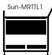
Sun-MRTTL1 98cm(H) 81cm(W) 52cm(D) 83cm(W) 57cm(D) with buffers
