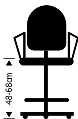
Sun-CHA4 Seat 46cm(W) 43cm(D) Width with arms 60cm Foot ring 46cm Ø Base 60cm Ø
