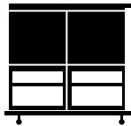
106cm(H) 121cm(W) 52cm(D) 121cm(W) 57cm(D) with buffers
