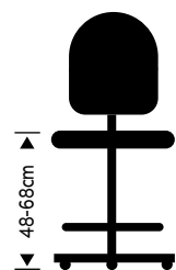
Sun-CHA3 Seat 46cm(W) 43cm(D) Foot ring 46cm Ø Base 60cm Ø
