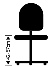
Sun-CHA1 Seat 46cm(W) 43cm(D) Base 60cm Ø
